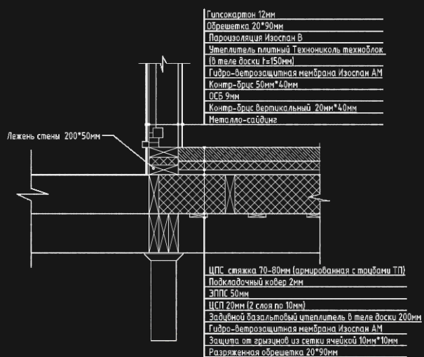
УЗЕЛ ПРИМЫКАНИЯ ТЕРРАСЫ
