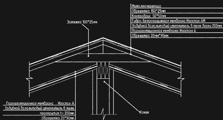
УЗЕЛ КОНЬКА КРЫШИ
