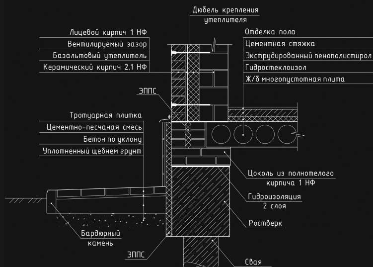
УЗЕЛ ПРИМЫКАНИЯ ПОЛА И ВНЕШНЕЙ СТЕНЫ
