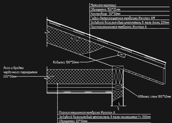
КОНСТРУКТИВНЫЙ УЗЕЛ СТОПИЛЬНОЙ СИСТЕМЫ
