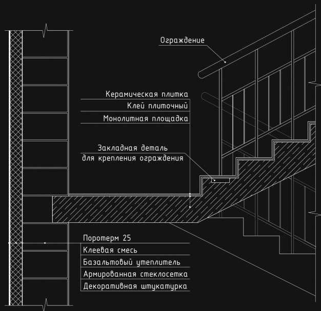
УЗЕЛ ПРИМЫКАНИЯ ЛЕСТНИЦЫ И ВНЕШНЕЙ СТЕНЫ
